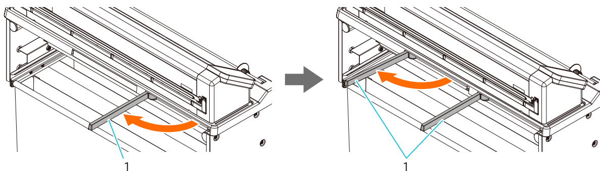
1. Stützstange
