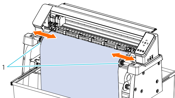
1. Flansche
