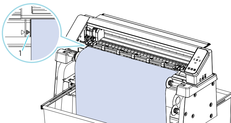
1. Indvendig retningslinje
